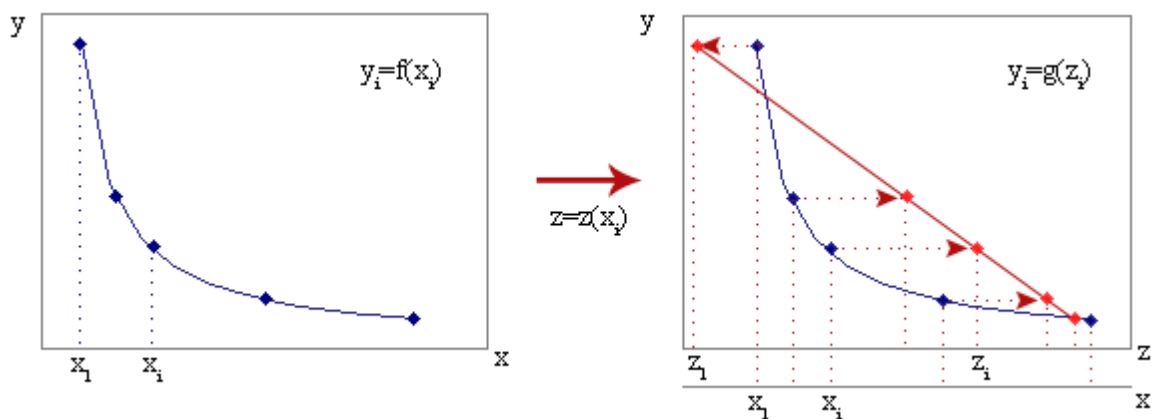
Рис.4. Графическое представление преобразования z=z(x) шкалы ценообразующего фактора x для линеаризации зависимости y=g(z) от преобразованных значений z фактора x
