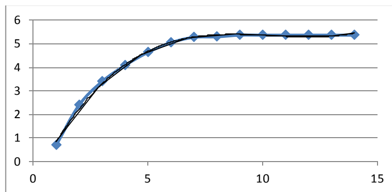
Рис.5. Пример выявленного с помощью макроса «Поиск решения» нелинейного преобразования значений X_{\text{преобр}}=f(X_{\text{исходн}}) влияющего фактора (а - до сглаживания, б - после сглаживания «вручную»)
