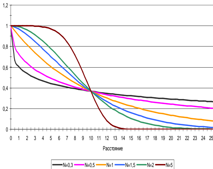
Рис.3. Графики параметрического семейства кривых, изменяющих вид в зависимости от параметра N
